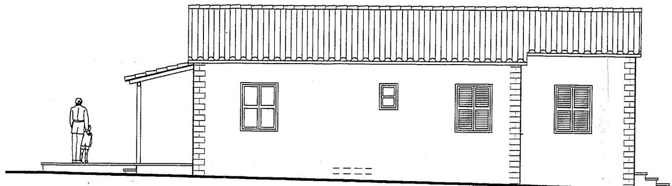
ΠΛΑΓΙΑ ΟΨΗ SIDE ELEVATION
