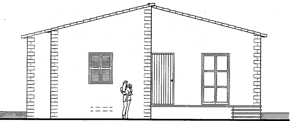
ΠΡΟΣΟΨΗ FRONT ELEVATION
